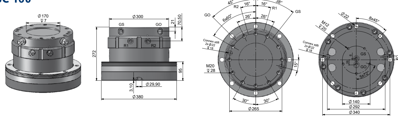
SC 160
