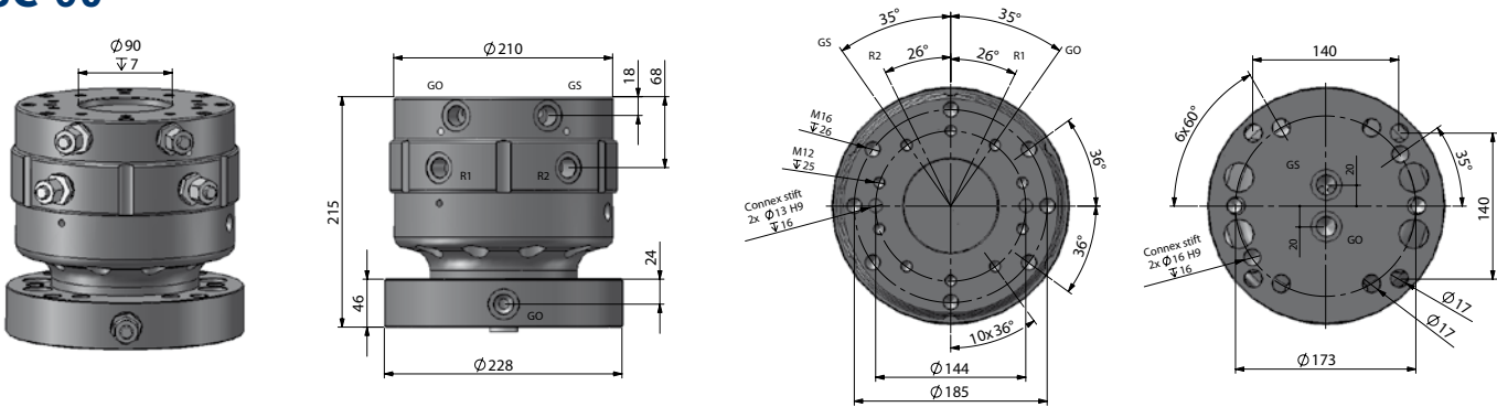
SC 60
