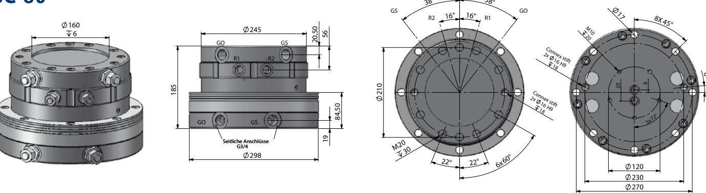
SC 80
