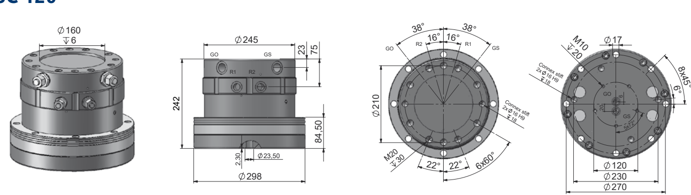
SC 120
